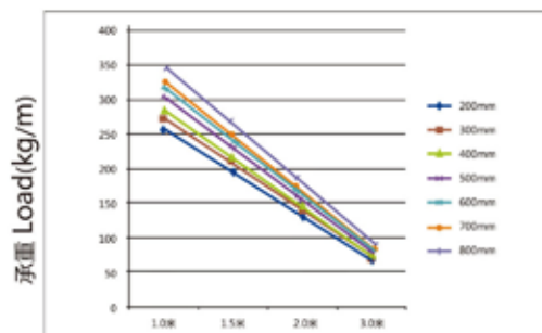
支撑间距 span
